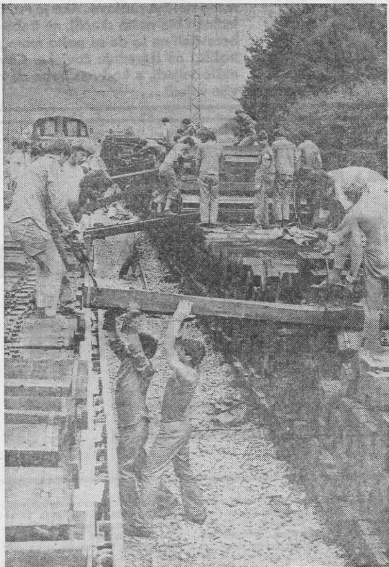
Istovari pragove, postavi ih, a po njima šine
