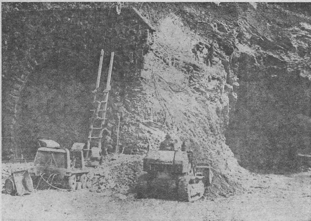
Dva kolosijeka — dva tunela, dvije kompozicije će juriti kroz srce planine
